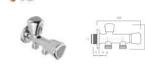
CODE: 301 20 02 00 Çift Çıkışlı Teherat Musluğu 1/2-1/2 Interval Tap 1/2-1/2 🔧 40 PCS.
